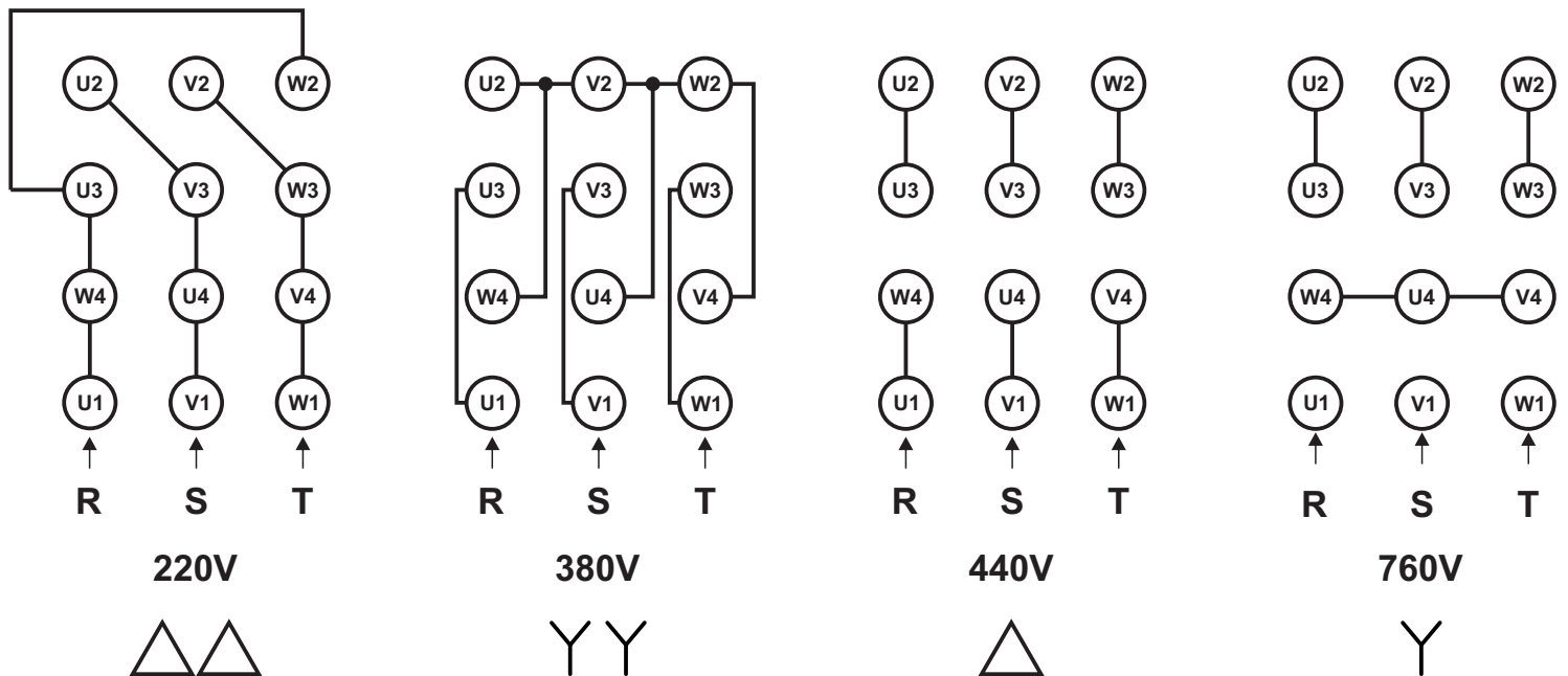
Ligação direta assíncrono
