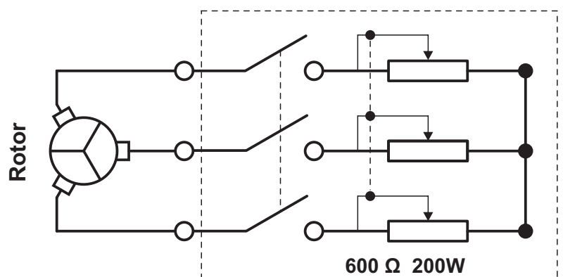
Chave e reostato externo
